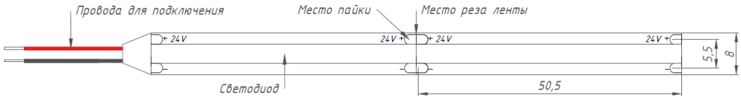
Рисунок 1 – Внешний вид светодиодной ленты COB.
